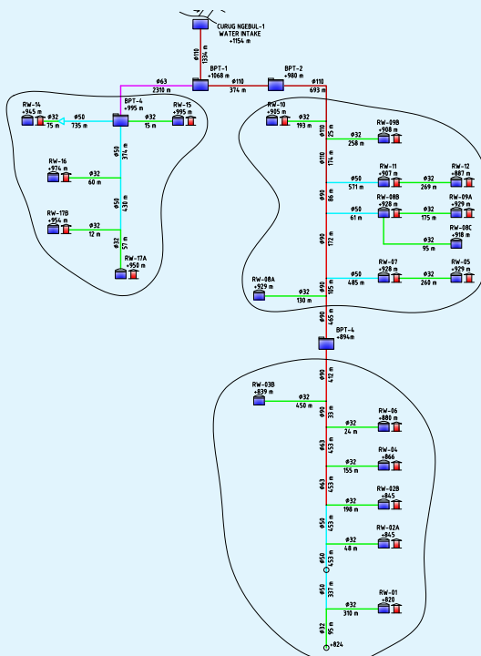
Schema watervoorziening
